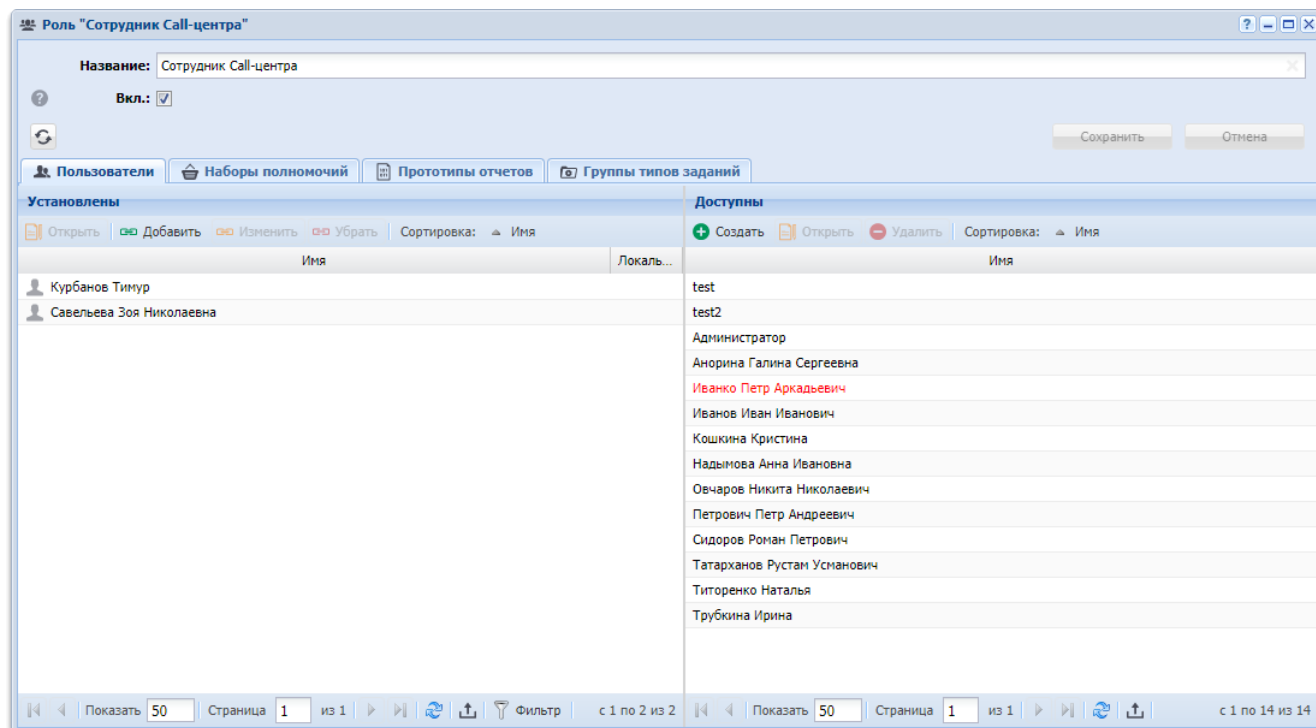
Рисунок 3.42. Модуль редактирования роли. Пример вкладки с таблицами «Установлены» и «Доступны»
