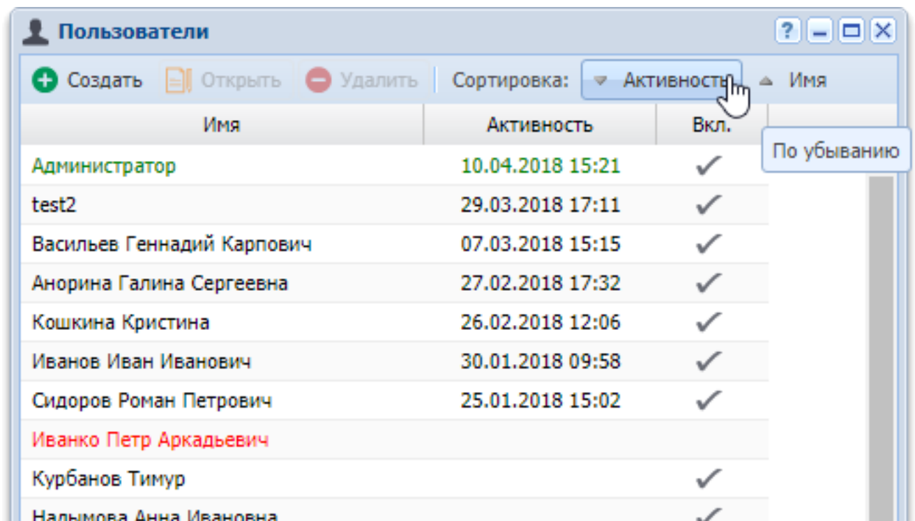
Рисунок 3.14. Кнопки для выполнения сортировки по столбцам «Активность» (по убыванию) и «Имя» (по возрастанию)
