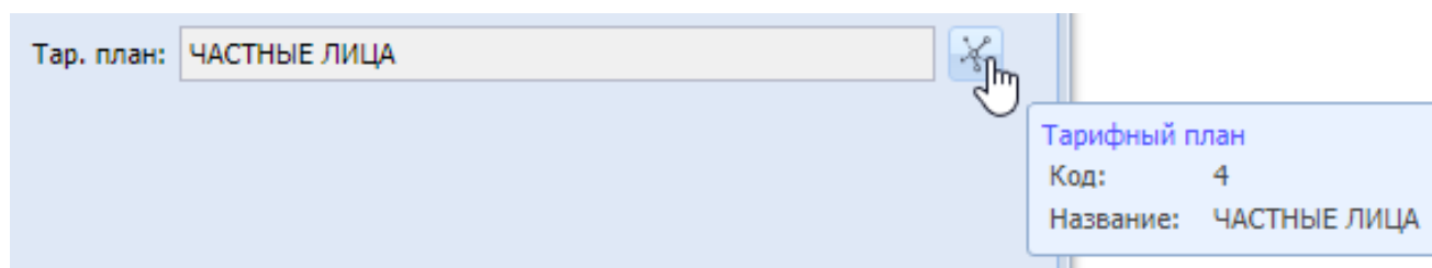
Рисунок 3.46. Поле выбора заблокировано от ввода, в нем указан тарифный план. Указатель мыши наведен на кнопку, предназначенную для открытия тарифного плана на просмотр и редактирование, отображается подсказка с информацией об этом тарифном плане
