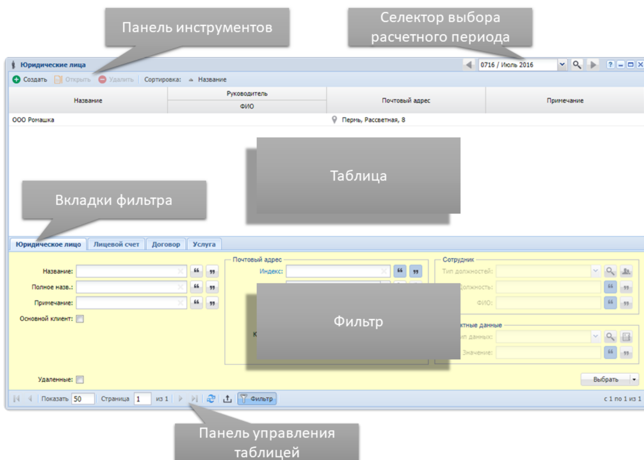
Рисунок 3.11. Поисковый модуль «Юридические лица»
