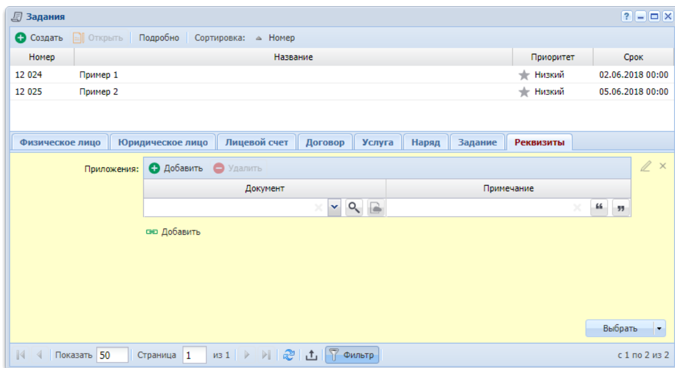
Рисунок 3.34. Поиск всех заданий, имеющих реквизит «Приложения»
