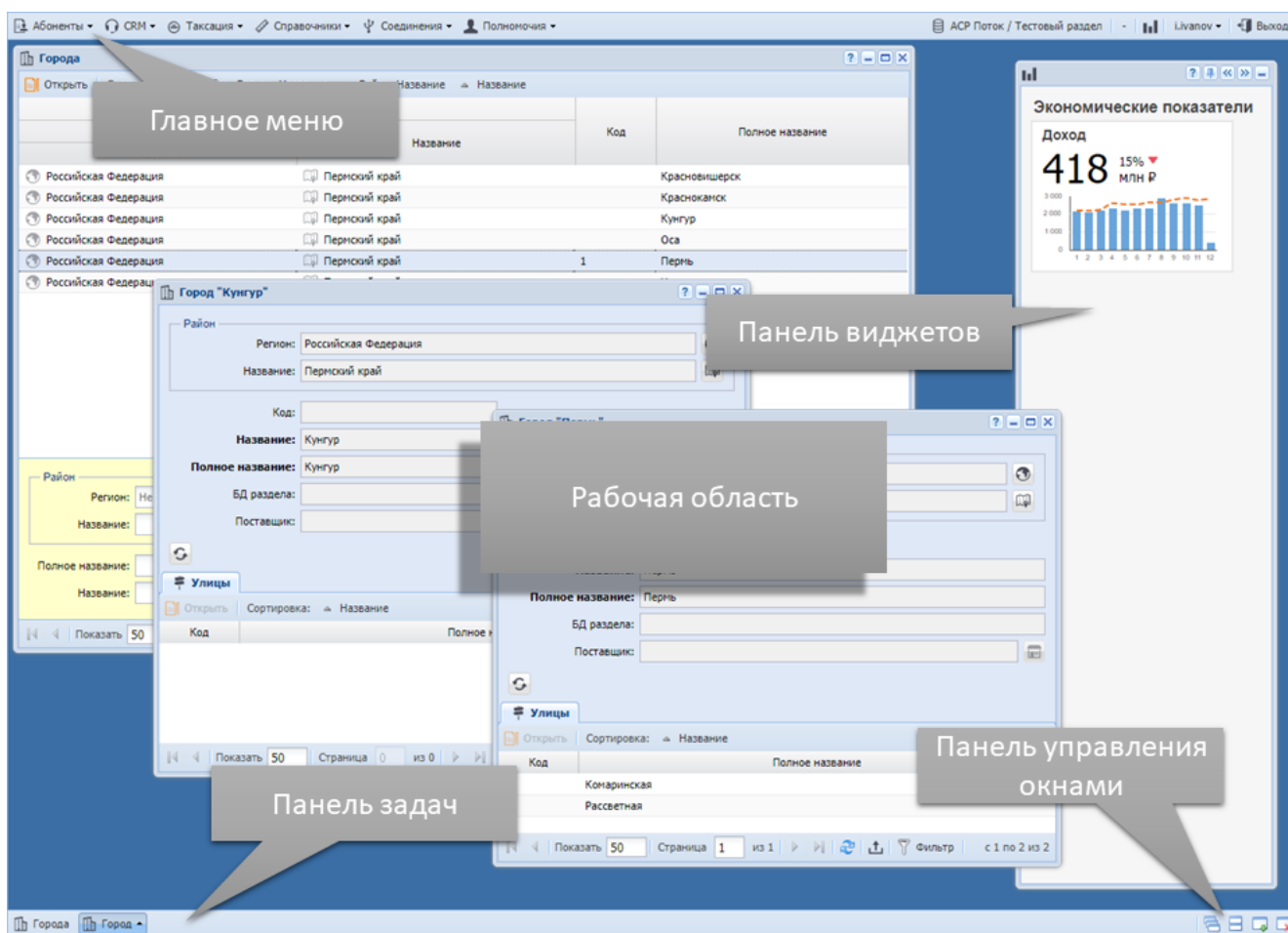
Рисунок 3.1. Главное окно системы
