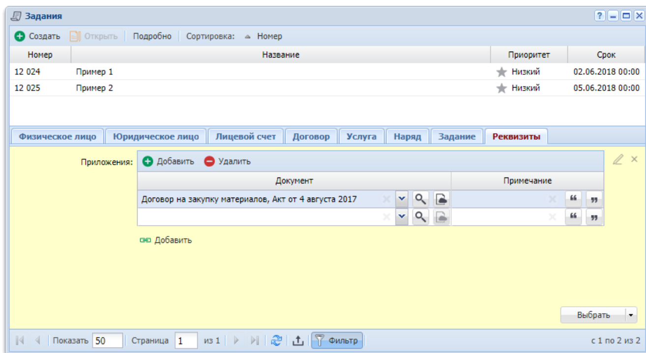
Рисунок 3.37. Поиск всех заданий, где в реквизите «Приложения» указан документ «Договор на закупку материалов» или документ «Акт от 4 августа 2017»
