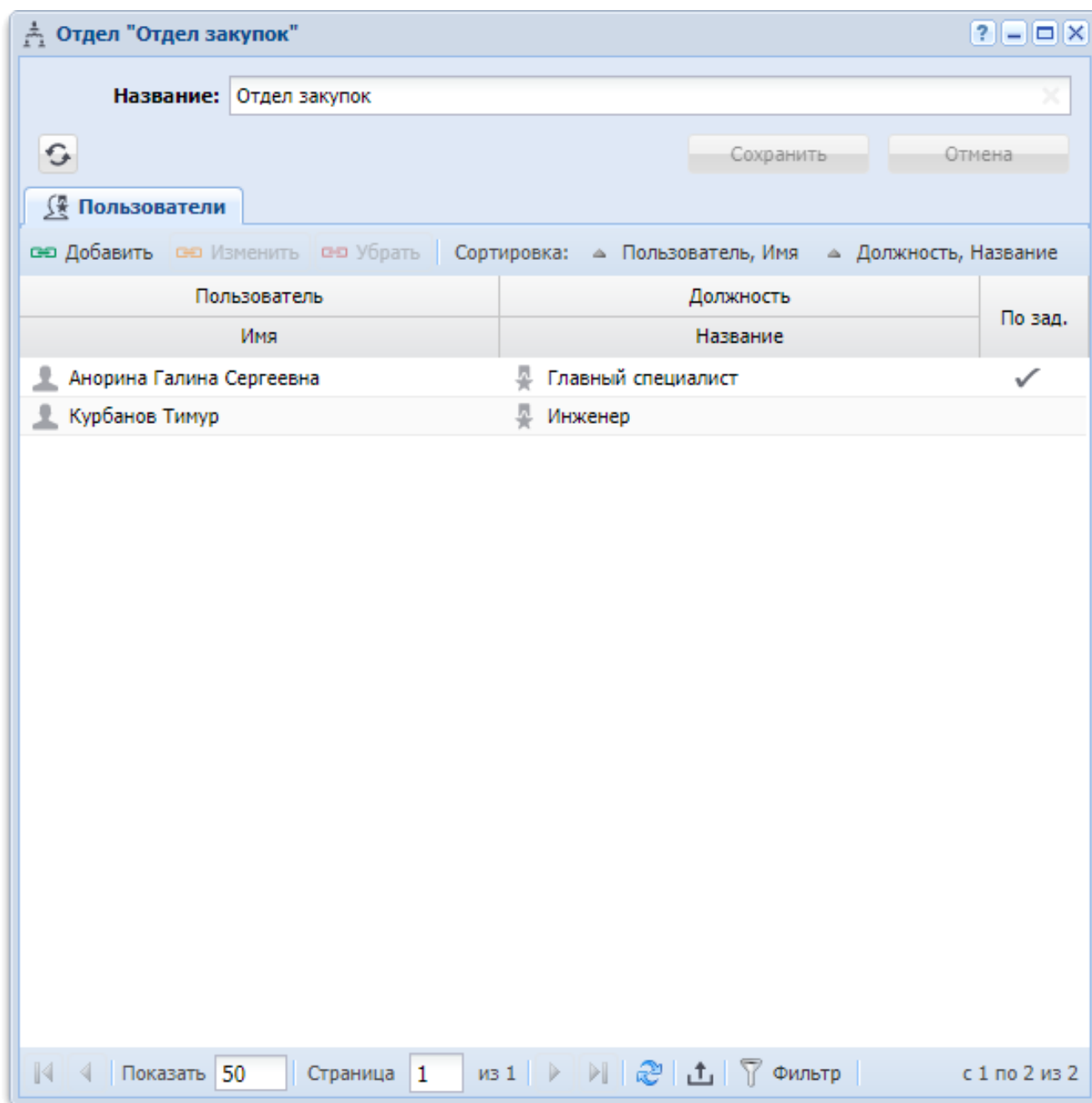
Рисунок 2.31. Модуль «Отдел»
