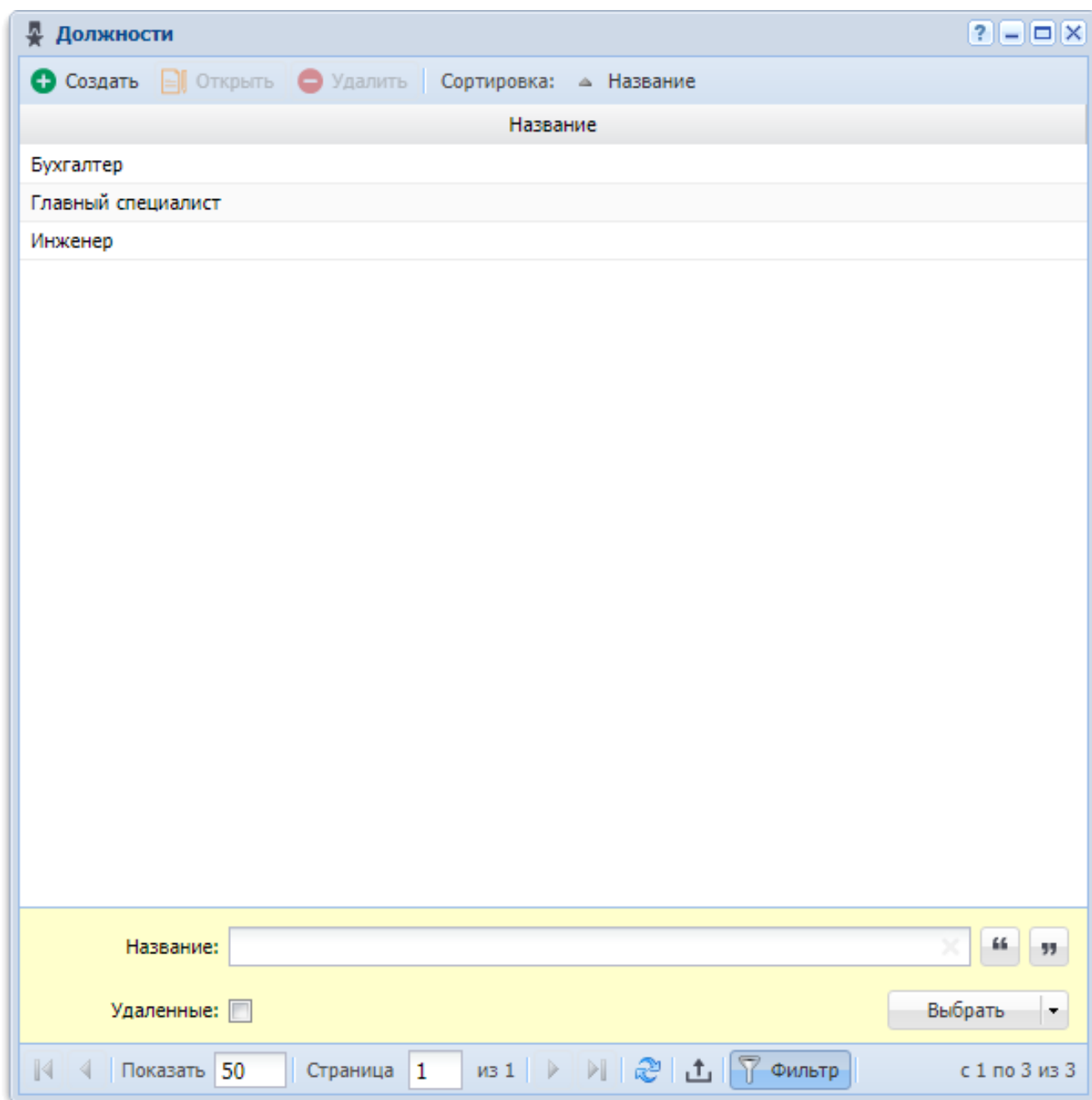
Рисунок 2.32. Модуль «Должности»
