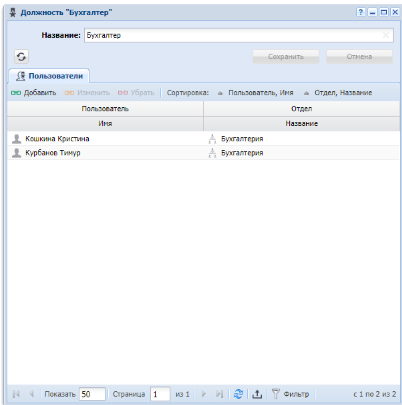
Рисунок 2.34. Модуль «Должность»
