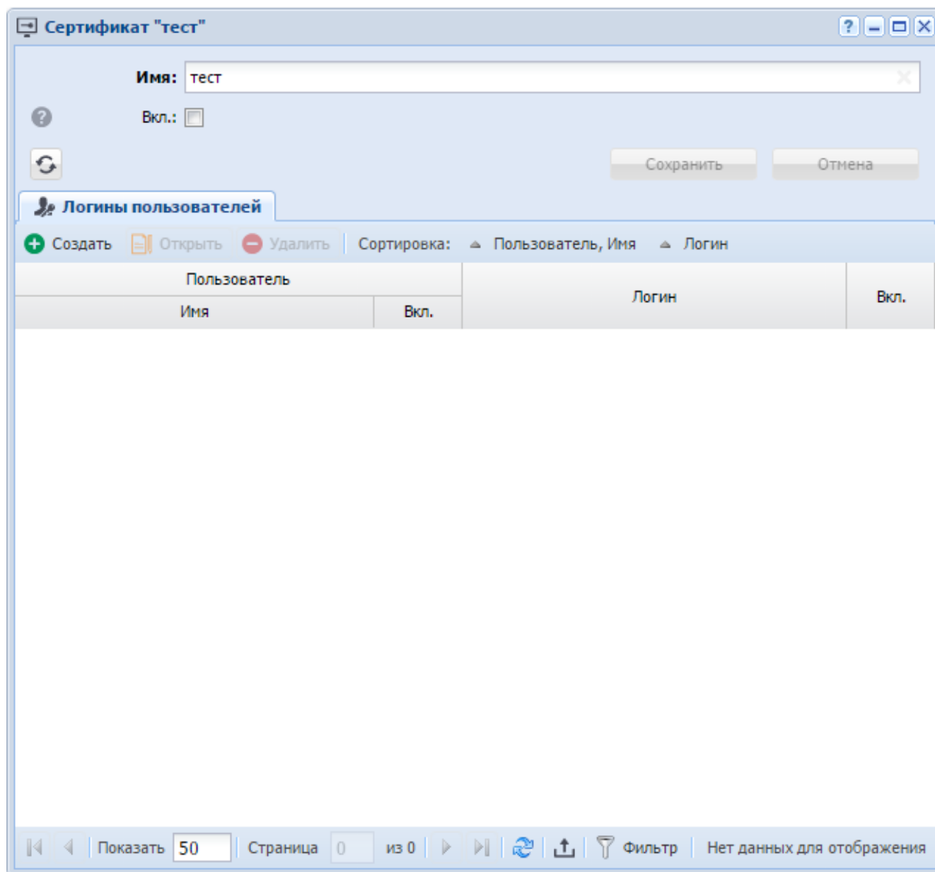
Рисунок 2.27. Модуль «Сертификат»
