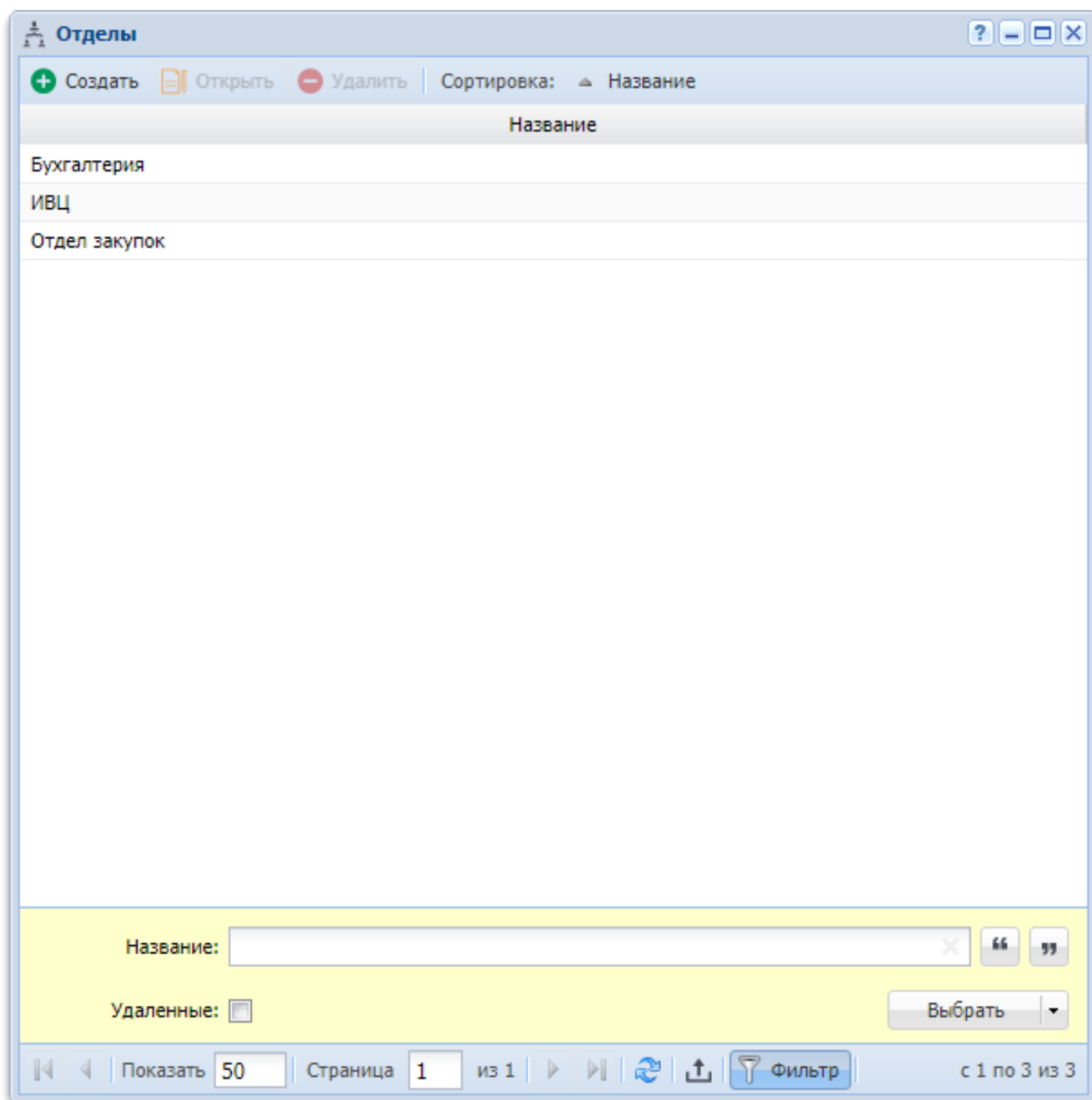
Рисунок 2.29. Модуль «Отделы»
