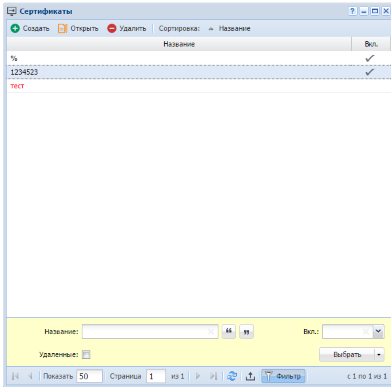
Рисунок 2.25. Модуль «Сертификаты»
