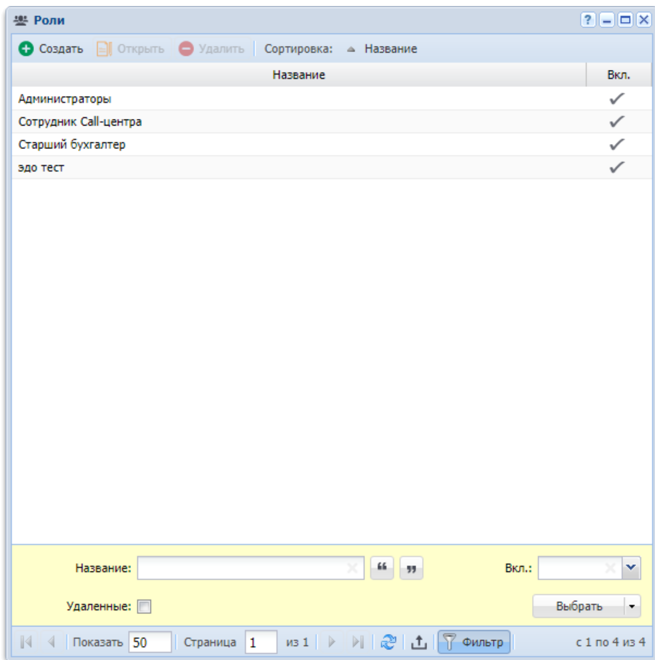
Рисунок 2.10. Модуль «Роли»
