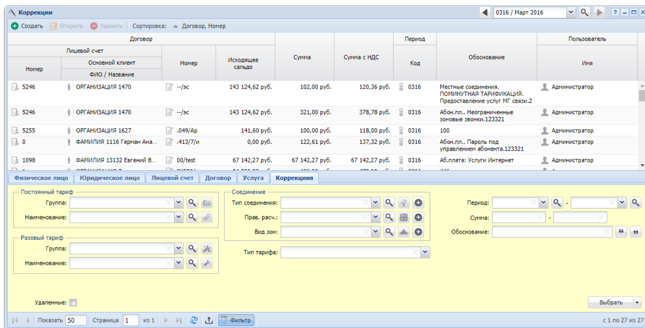
Рисунок 2.24. Модуль «Коррекции»
