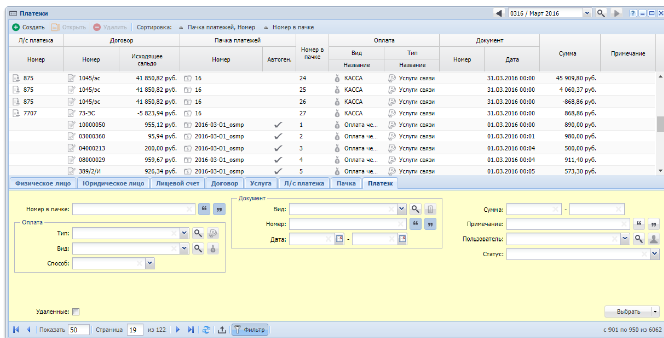
Рисунок 2.14. Модуль «Платежи»
