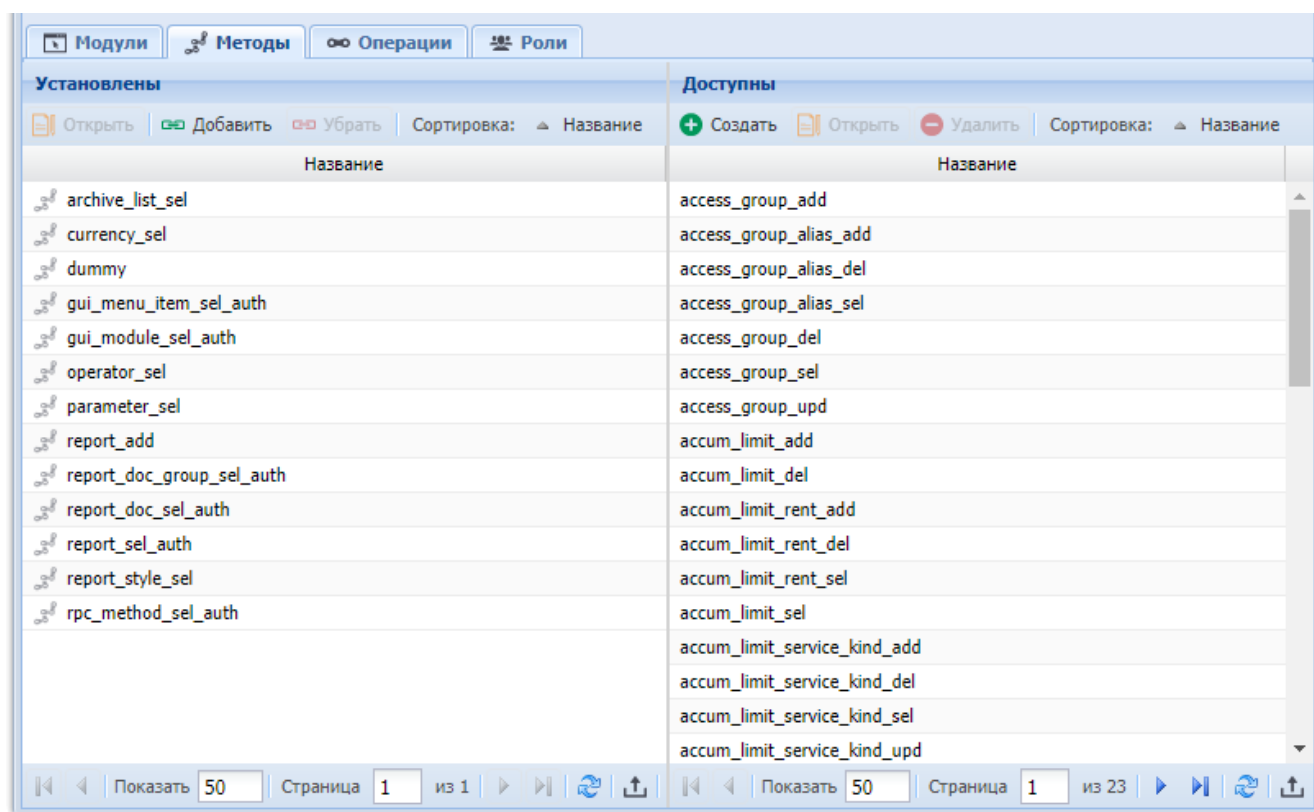
Рисунок 2.23. Модуль «Набор полномочий», фрагмент. Вкладка «Методы»
