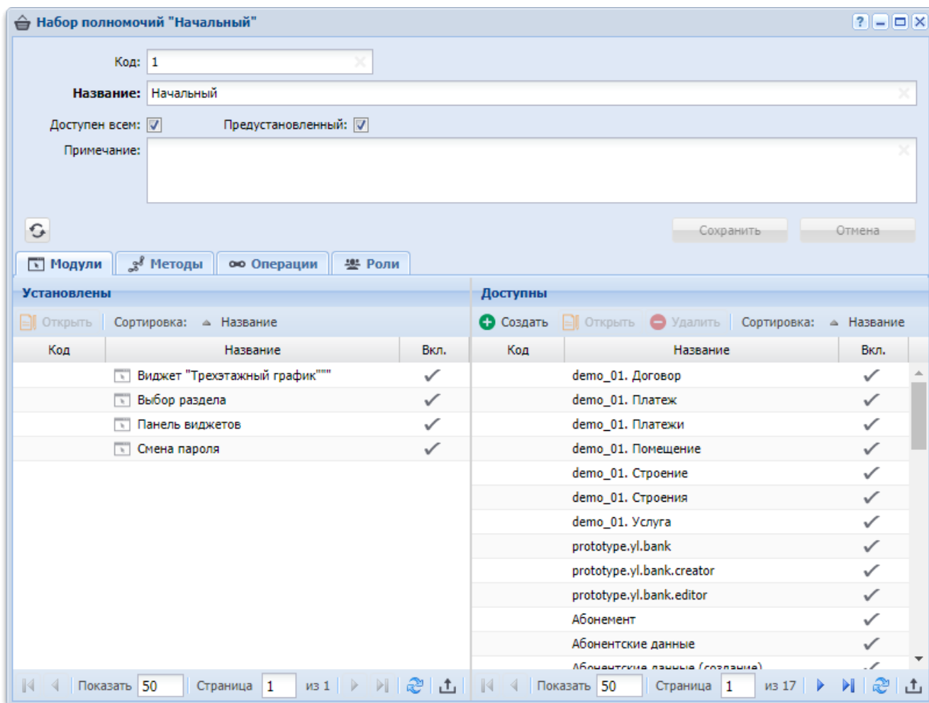
Рисунок 2.22. Модуль «Набор полномочий». Вкладка «Модули»
