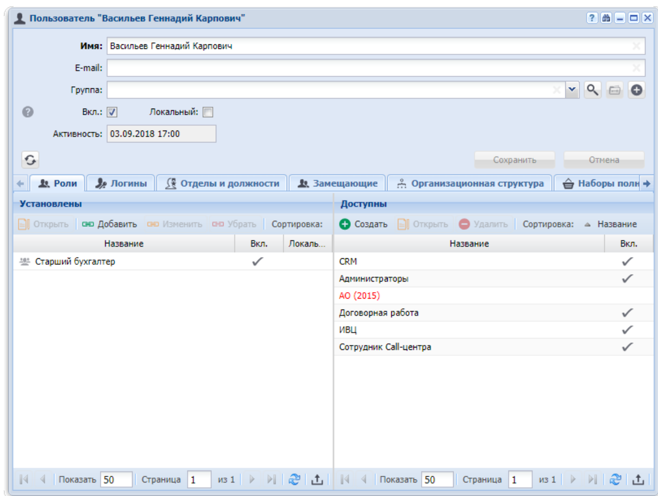
Рисунок 2.3. Модуль «Пользователь». Вкладка «Роли»
