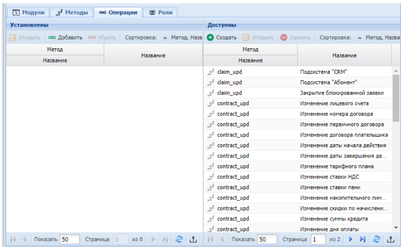
Рисунок 2.24. Модуль «Набор полномочий», фрагмент. Вкладка «Операции»
