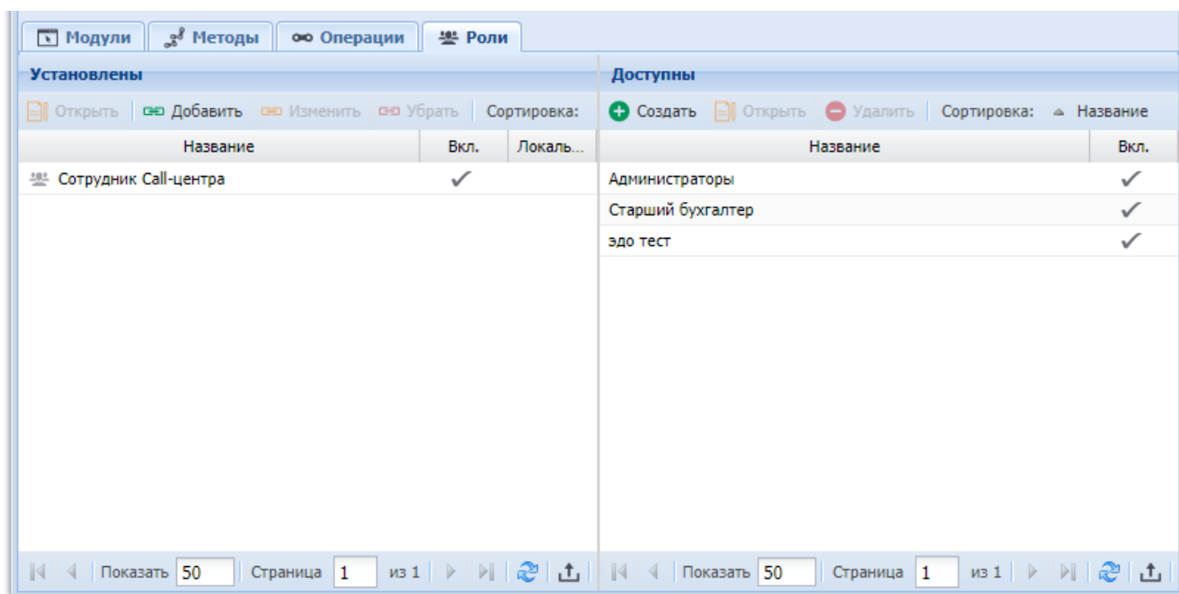
Рисунок 2.25. Модуль «Набор полномочий», фрагмент. Вкладка «Роли»
