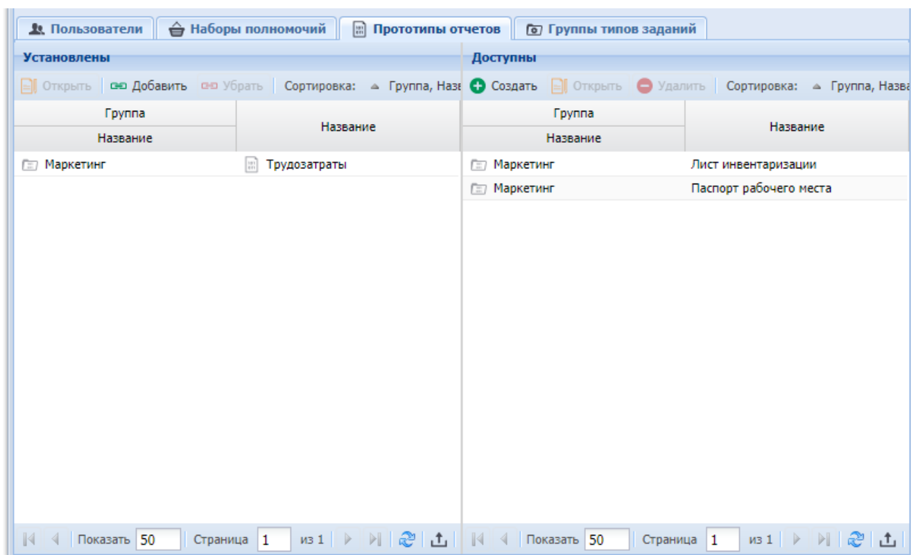
Рисунок 2.15. Модуль «Роль». Вкладка «Прототипы отчетов»
