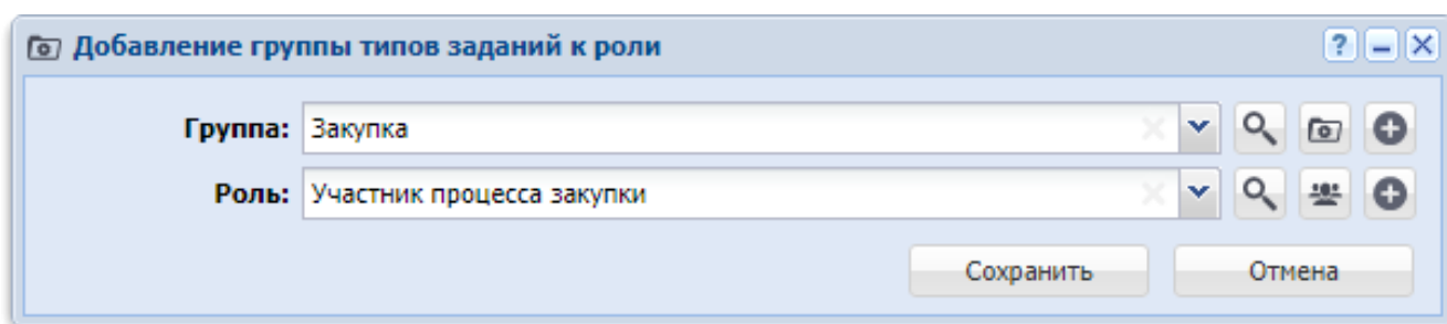
Рисунок 3.2. Модуль «Добавление группы типов заданий к роли»
