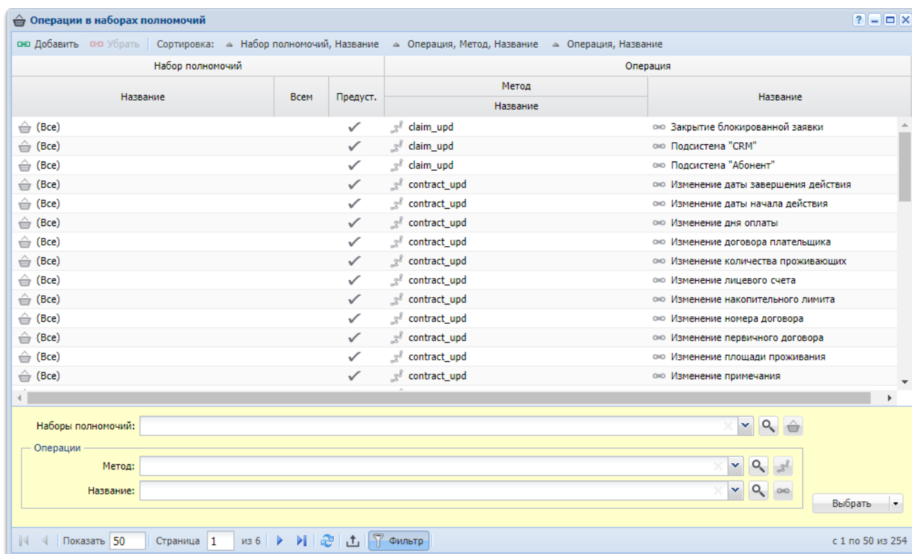
Рисунок 3.16. Модуль «Операции в наборах полномочий»
