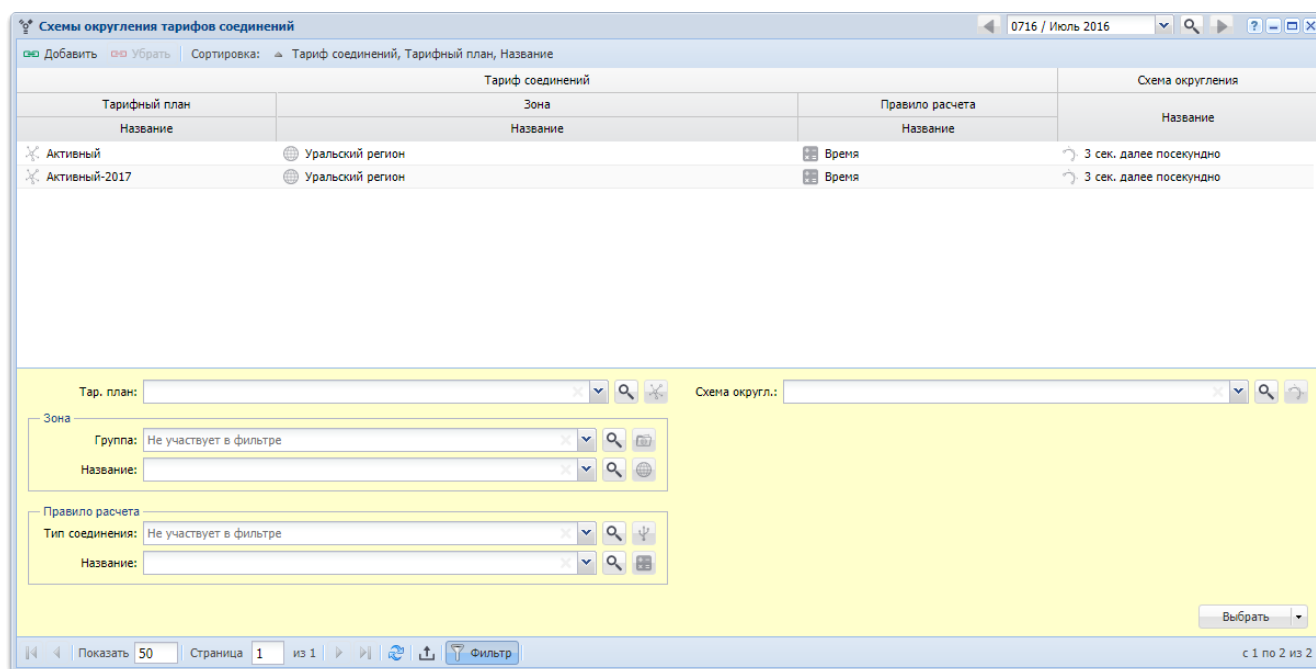
Рисунок 4.32. Модуль «Схемы округления тарифов соединений»
