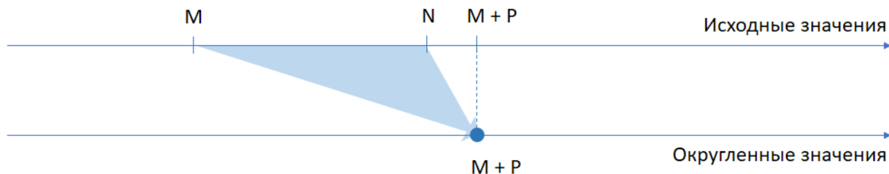
Рисунок 3.47. Округление в большую сторону. Шаг больше длины диапазона. (Округление до значения, большего верхней границы диапазона.)
