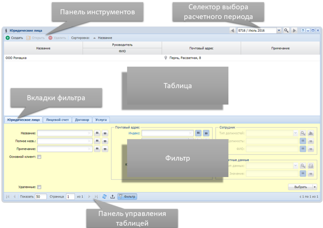
Рисунок 3.11. Поисковый модуль «Юридические лица»
